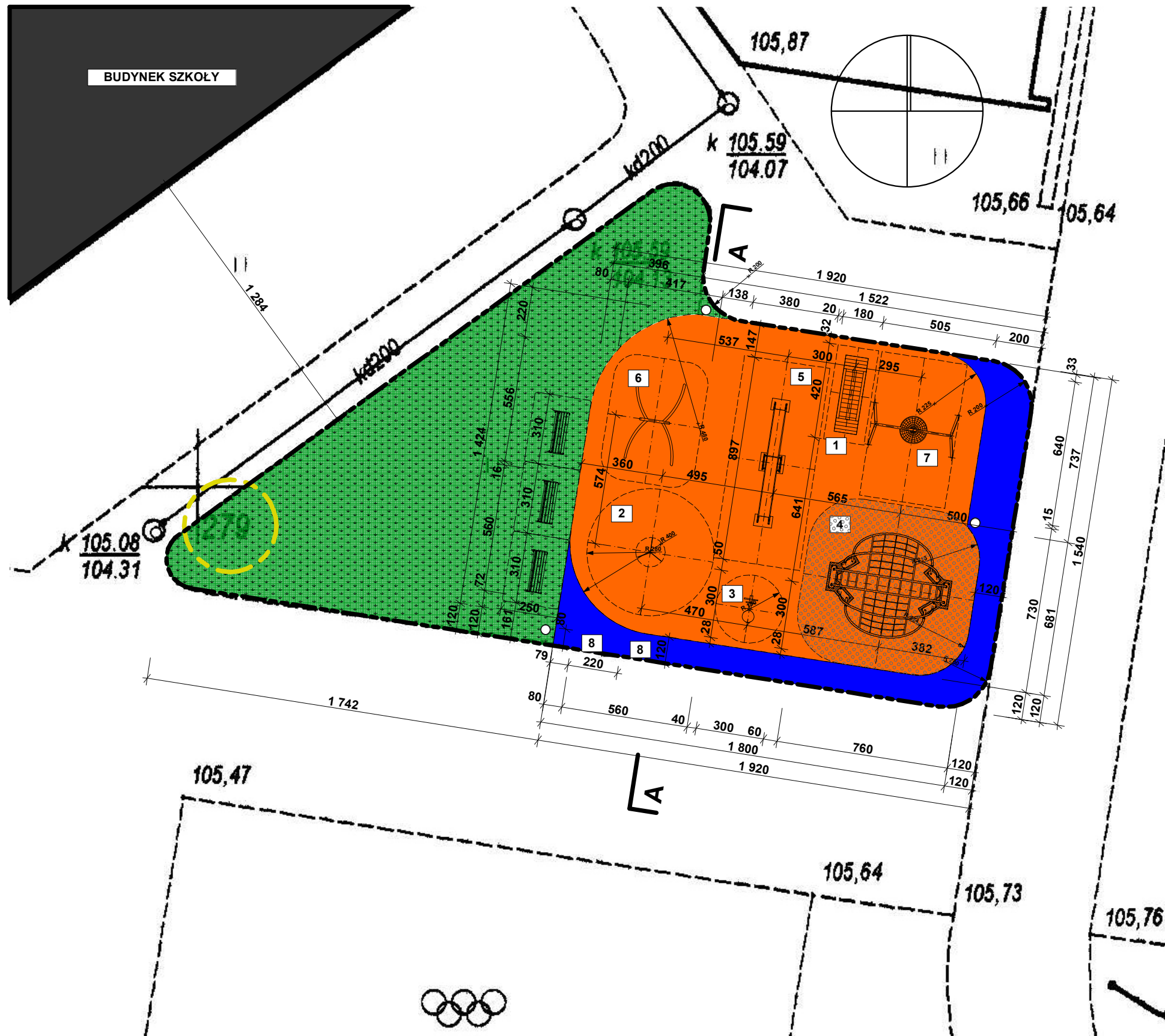
ZAGOSPODAROWANIE TERENU SKALA 1:200
